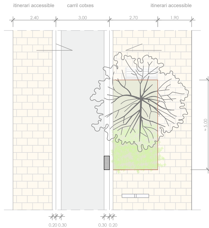
PLANTA TIPUS PROPOSTA
