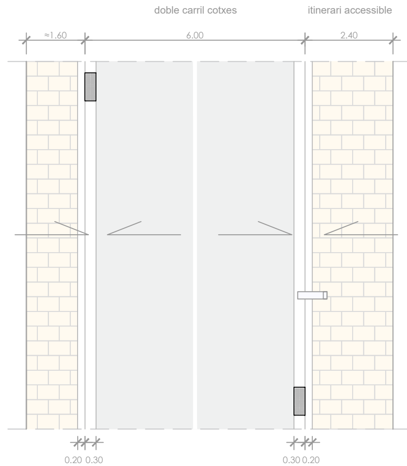
PLANTA TIPUS PROPOSTA
