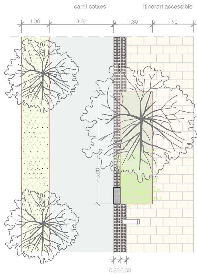
PLANTA TIPUS PROPOSTA
