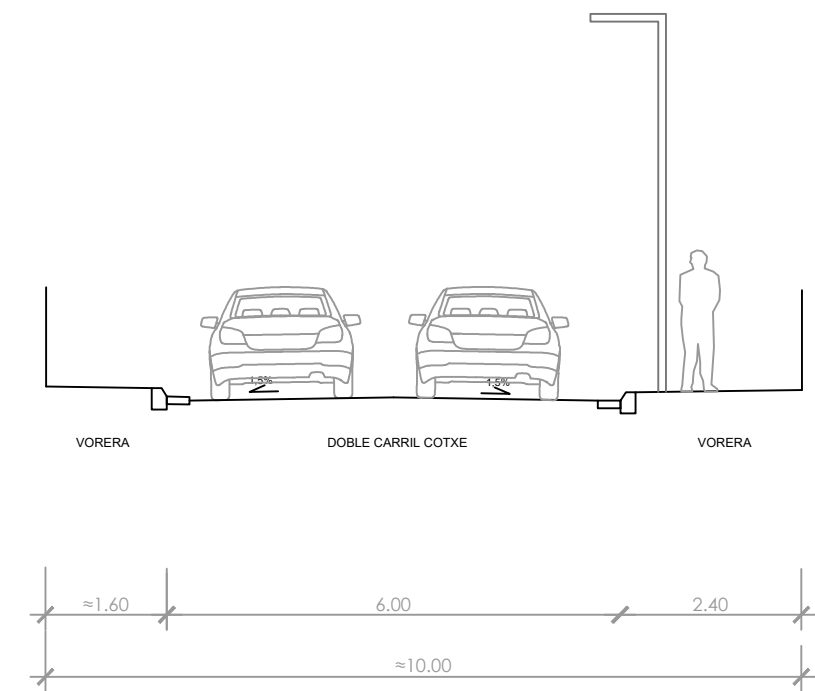
SECCIÓ PROPOSTA CARRER
