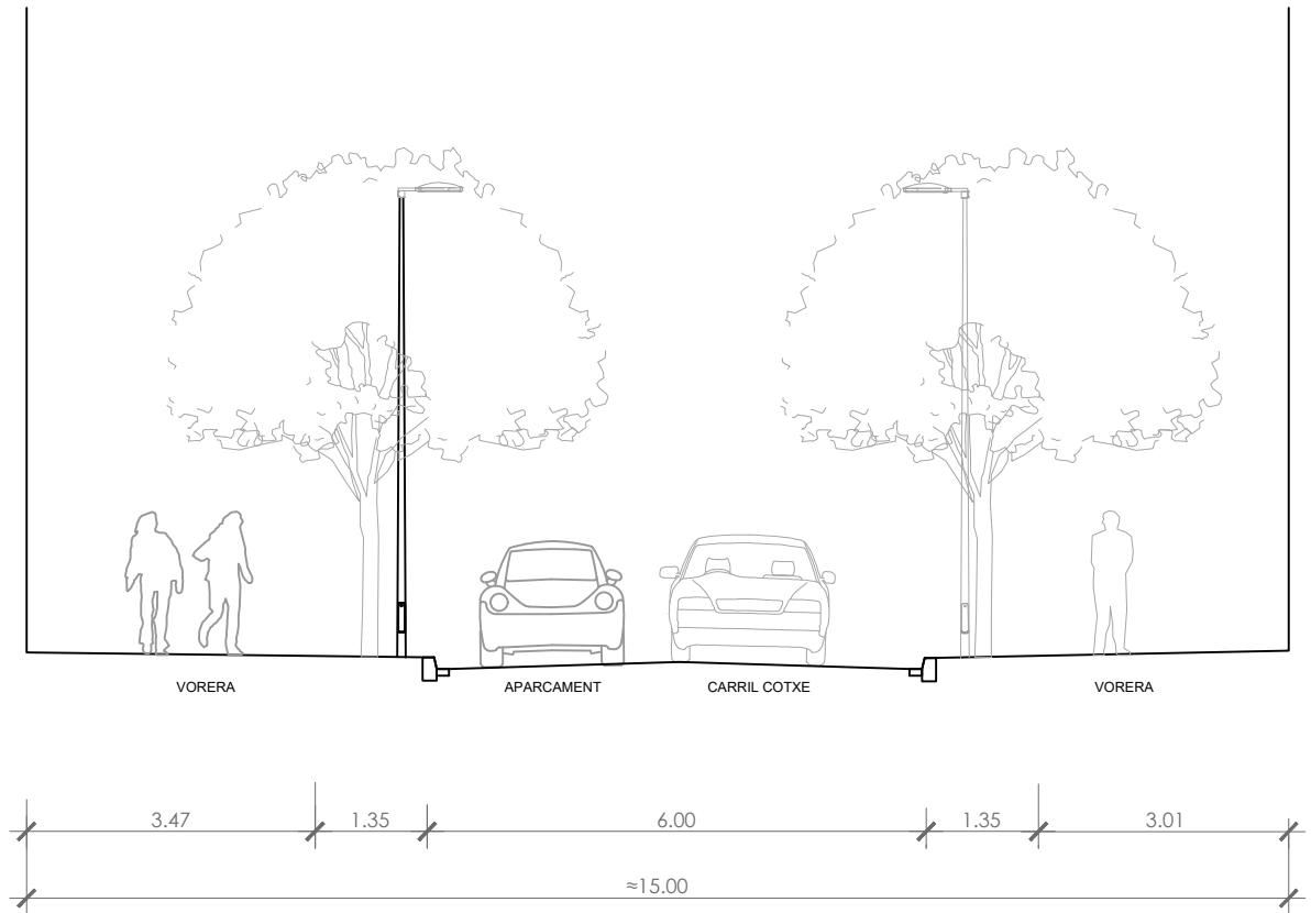
SECCIÓ ESTAT ACTUAL CARRER
