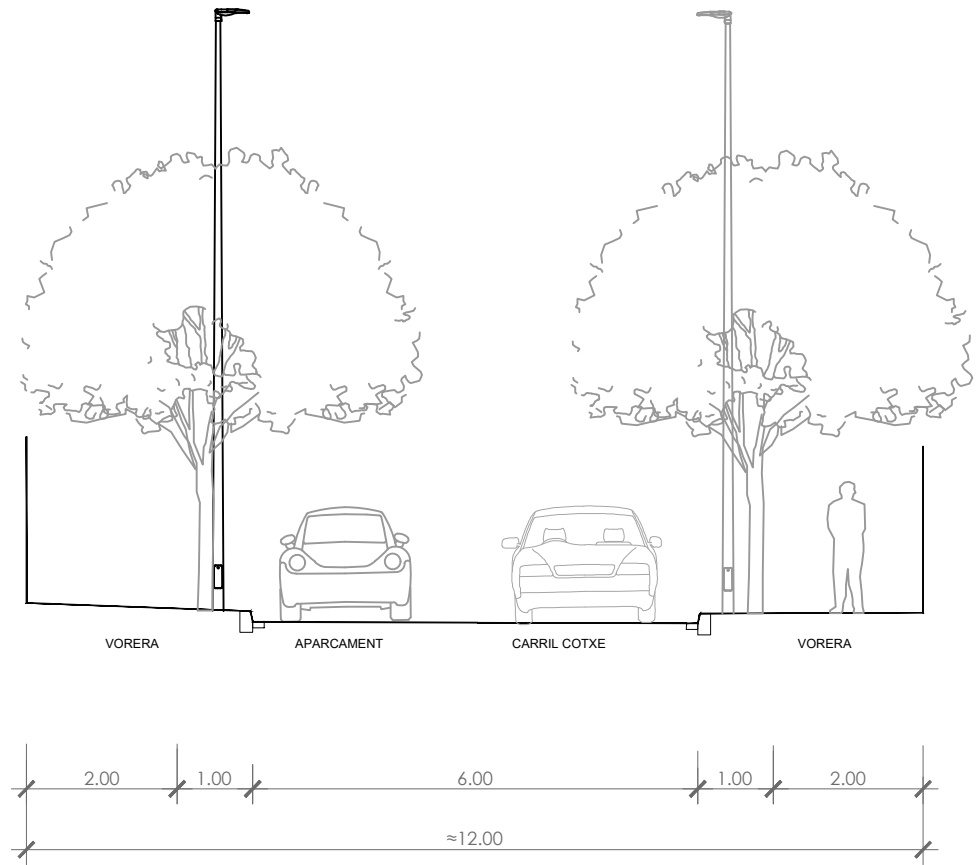
SECCIÓ ESTAT ACTUAL CARRER
