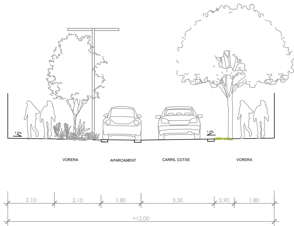
SECCIÓ PROPOSTA CARRER
