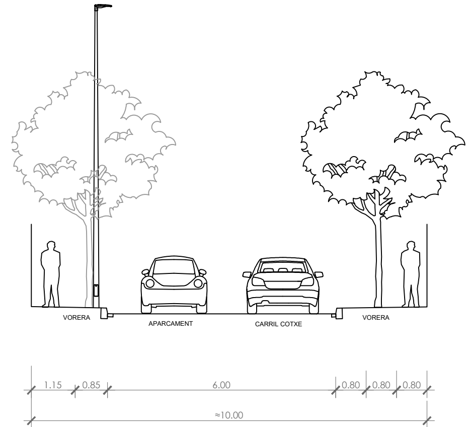
SECCIÓ ESTAT ACTUAL CARRER
