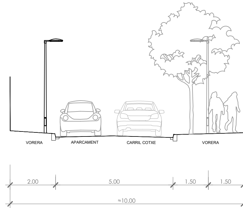
SECCIÓ ESTAT ACTUAL CARRER
