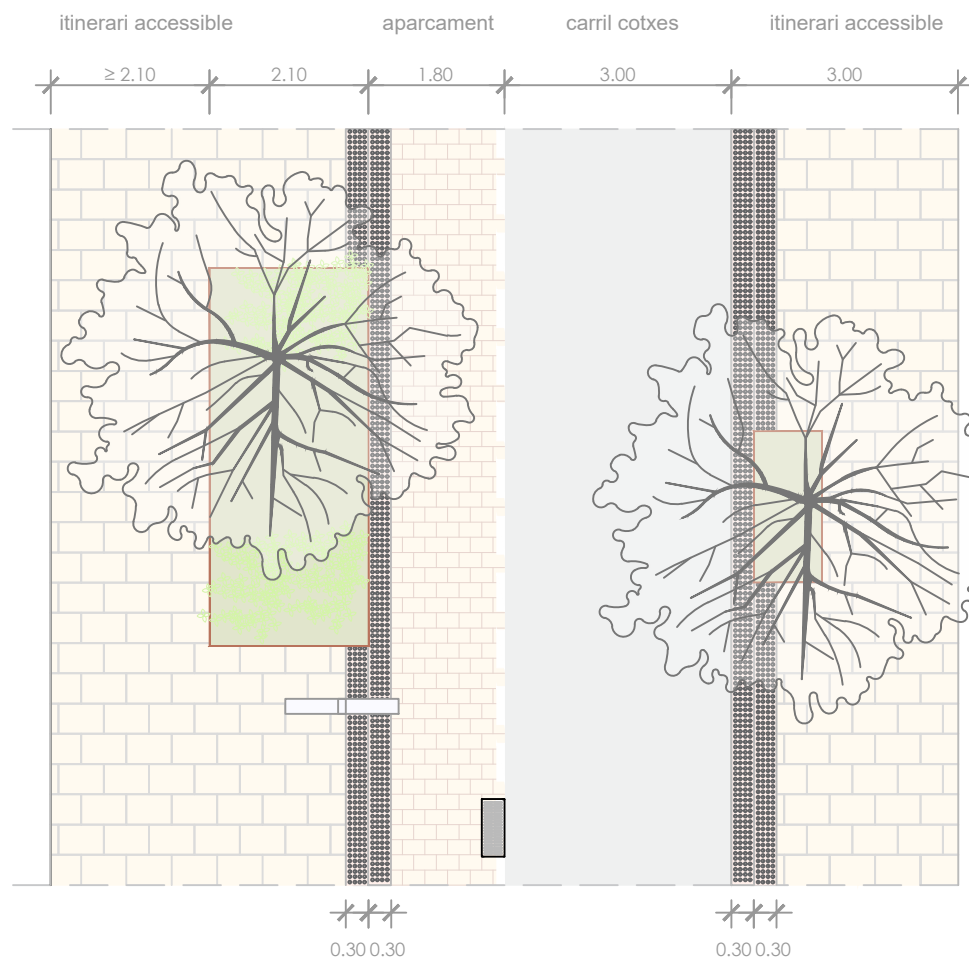
PLANTA TIPUS PROPOSTA
