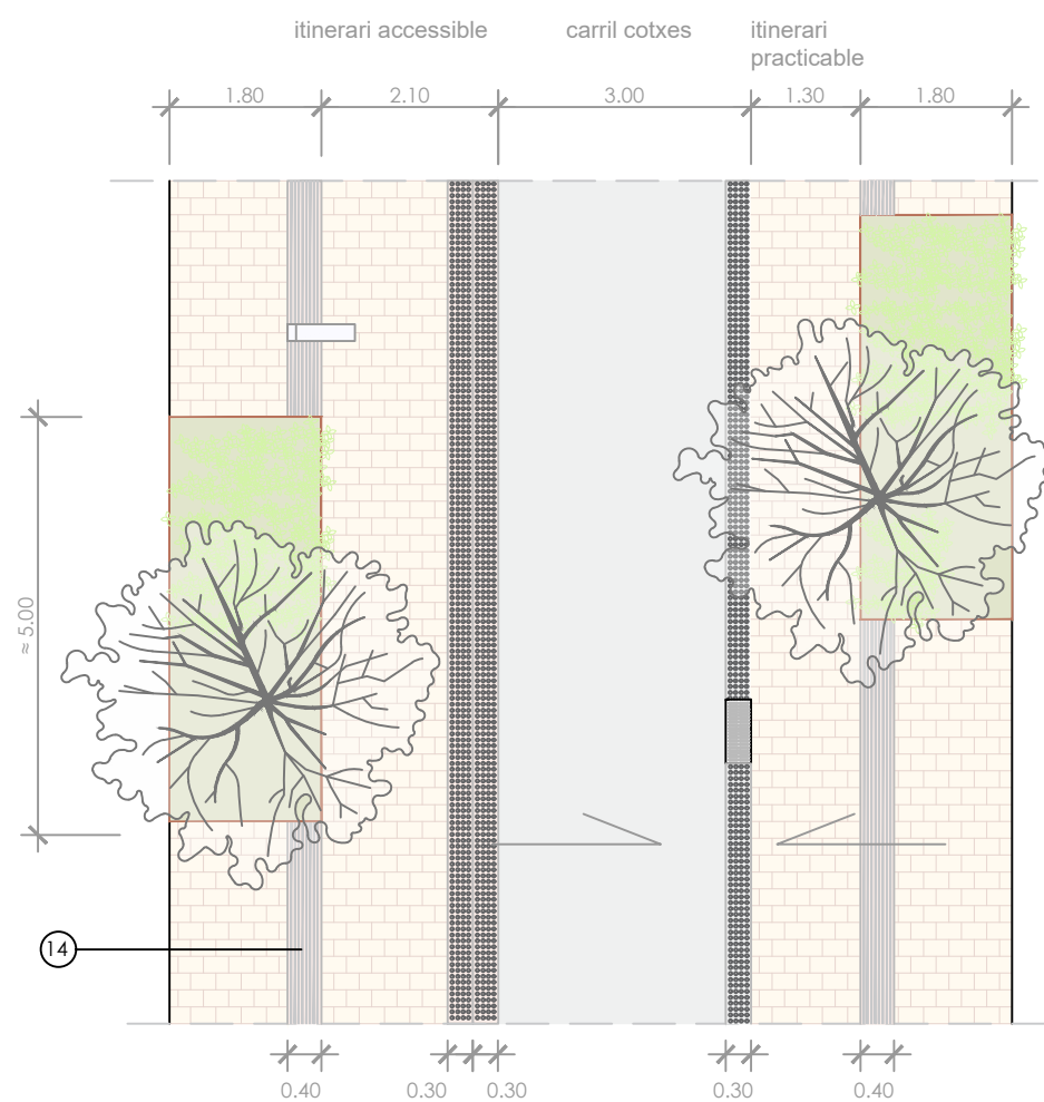
PLANTA TIPUS PROPOSTA
