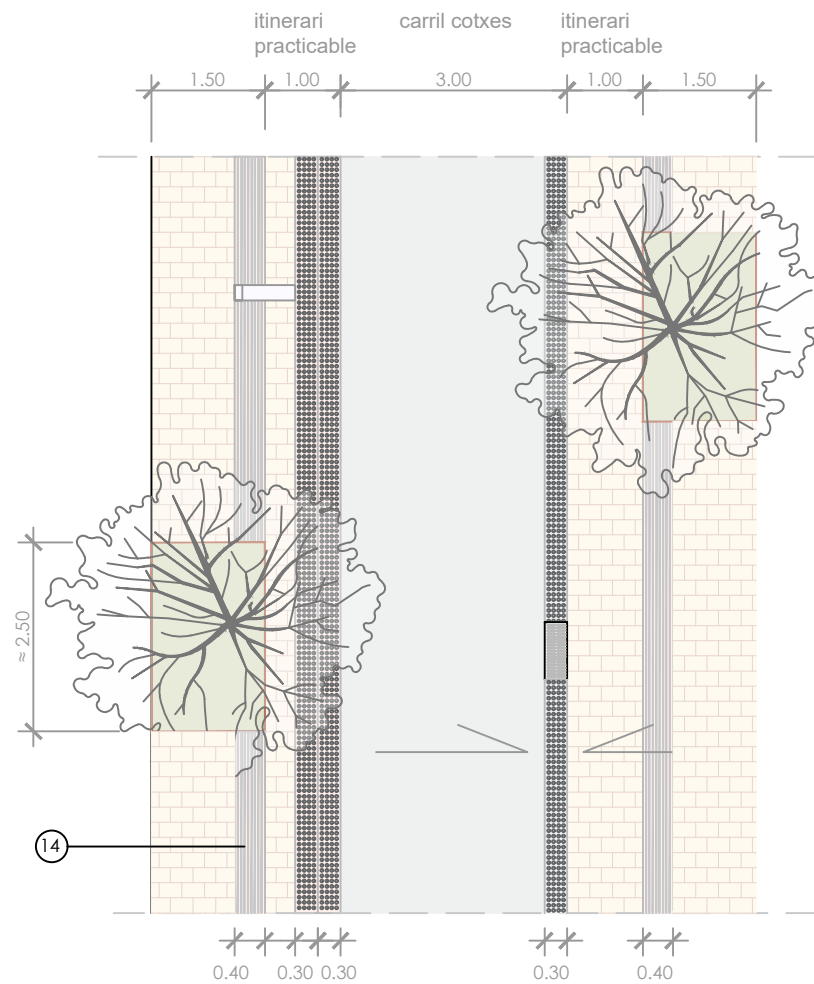
PLANTA TIPUS PROPOSTA
