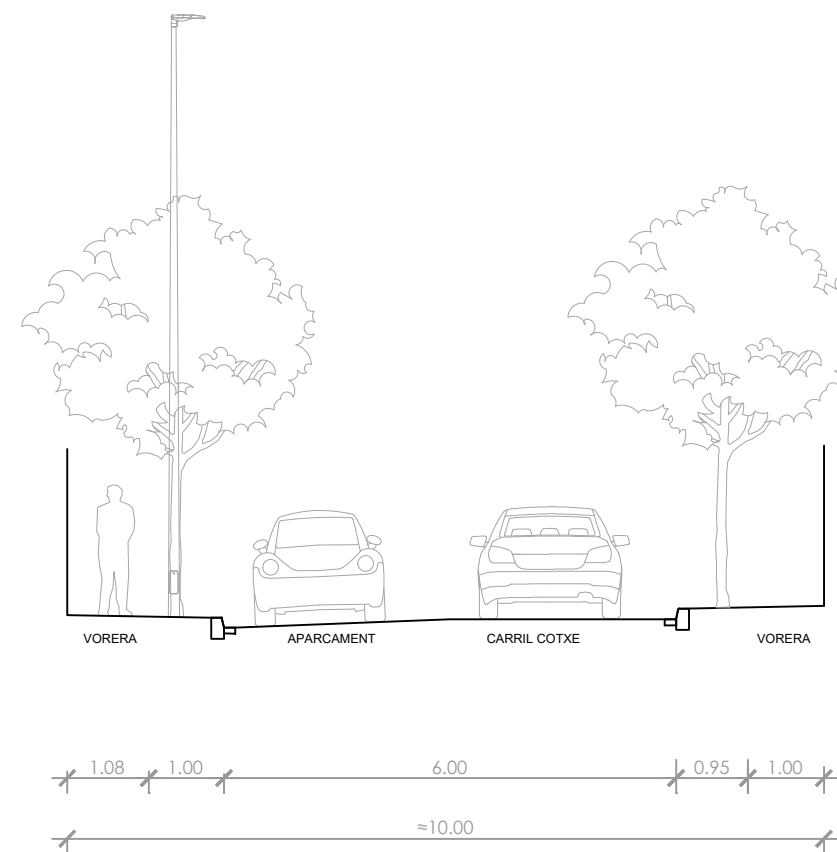
SECCIÓ ESTAT ACTUAL CARRER
