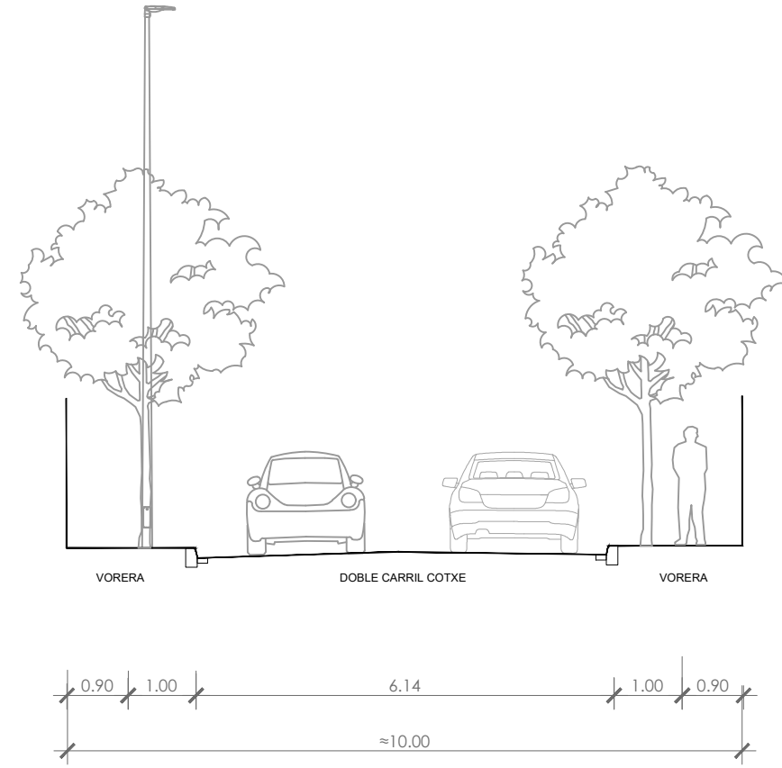
SECCIÓ ESTAT ACTUAL CARRER
