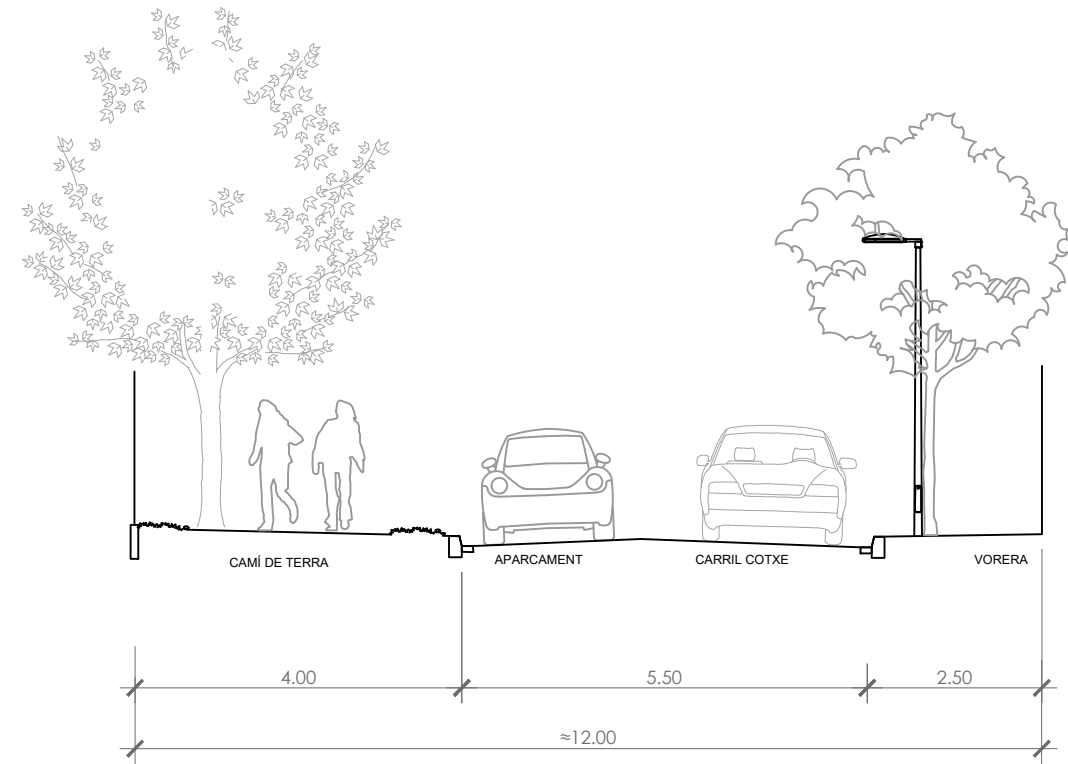
SECCIÓ ESTAT ACTUAL CARRER
