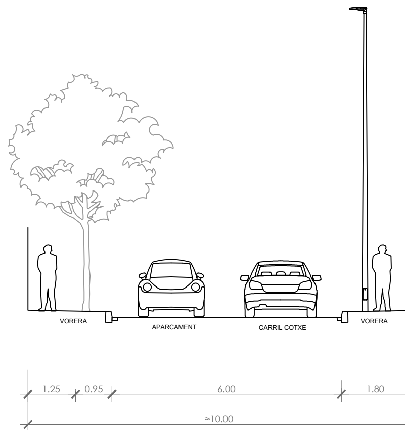
SECCIÓ ESTAT ACTUAL CARRER
