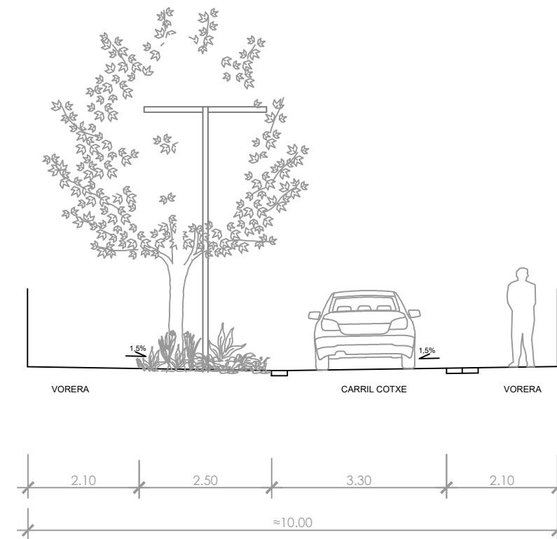
SECCIÓ PROPOSTA CARRER
