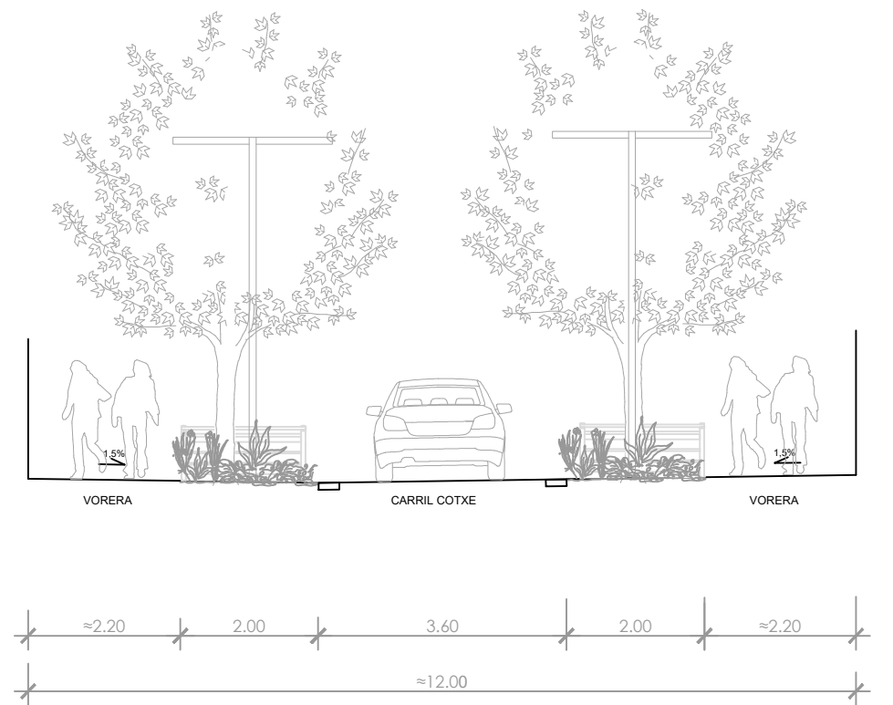
SECCIÓ PROPOSTA CARRER
