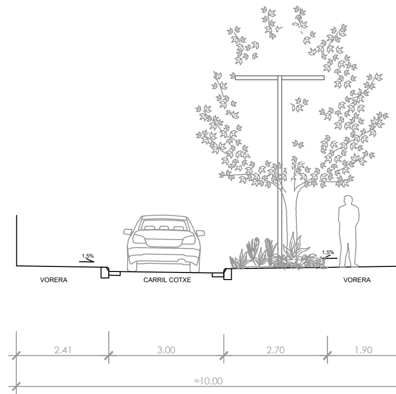
SECCIÓ PROPOSTA CARRER
