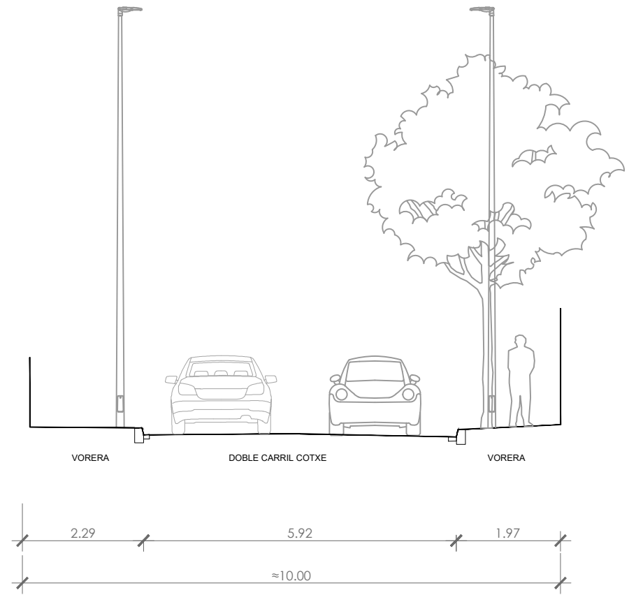
SECCIÓ ESTAT ACTUAL CARRER
