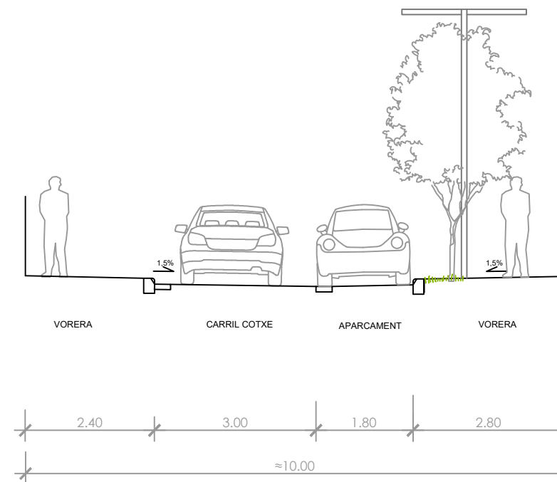
SECCIÓ PROPOSTA CARRER
