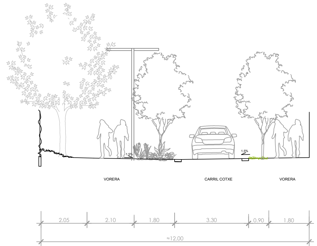
SECCIÓ ESTAT ACTUAL CARRER
