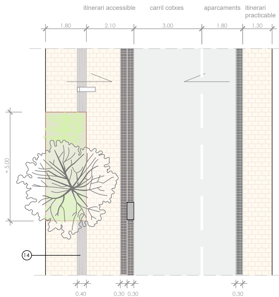
PLANTA TIPUS PROPOSTA C/ DE LA MINA
