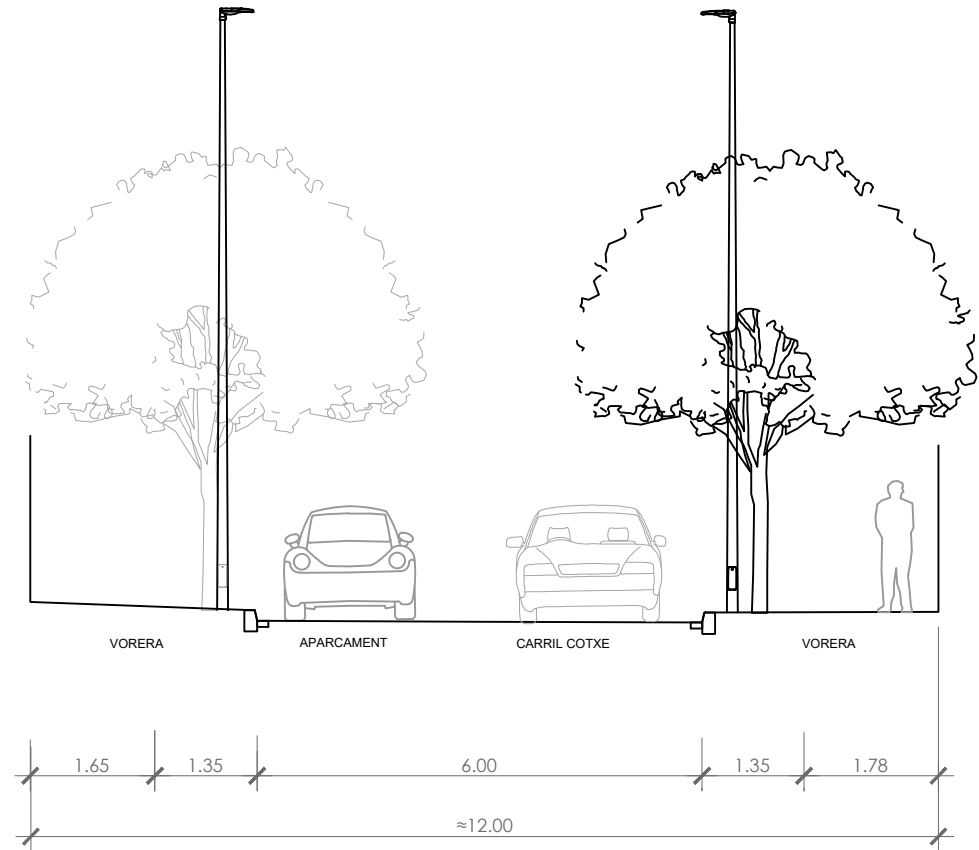
SECCIÓ ESTAT ACTUAL CARRER
