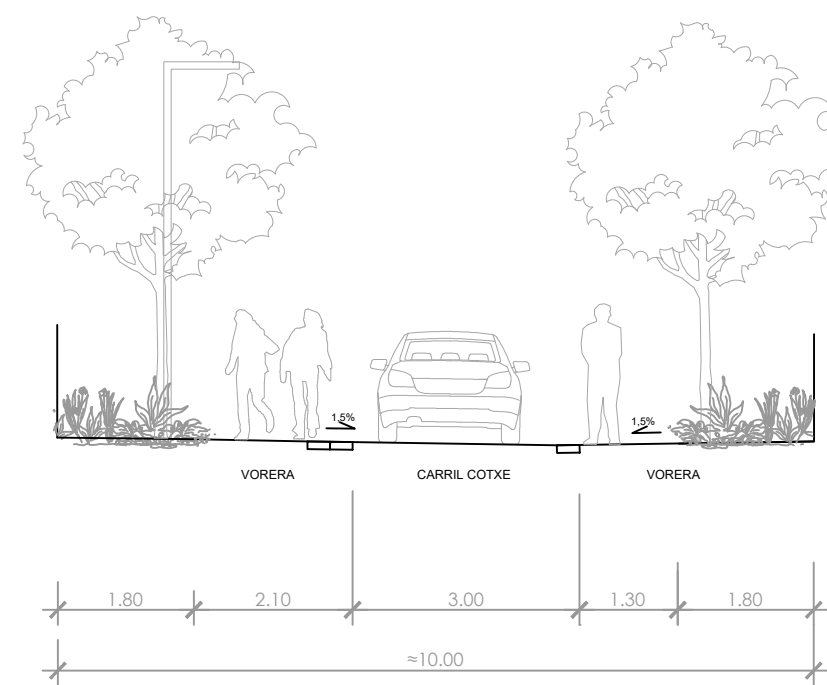
SECCIÓ PROPOSTA CARRER
