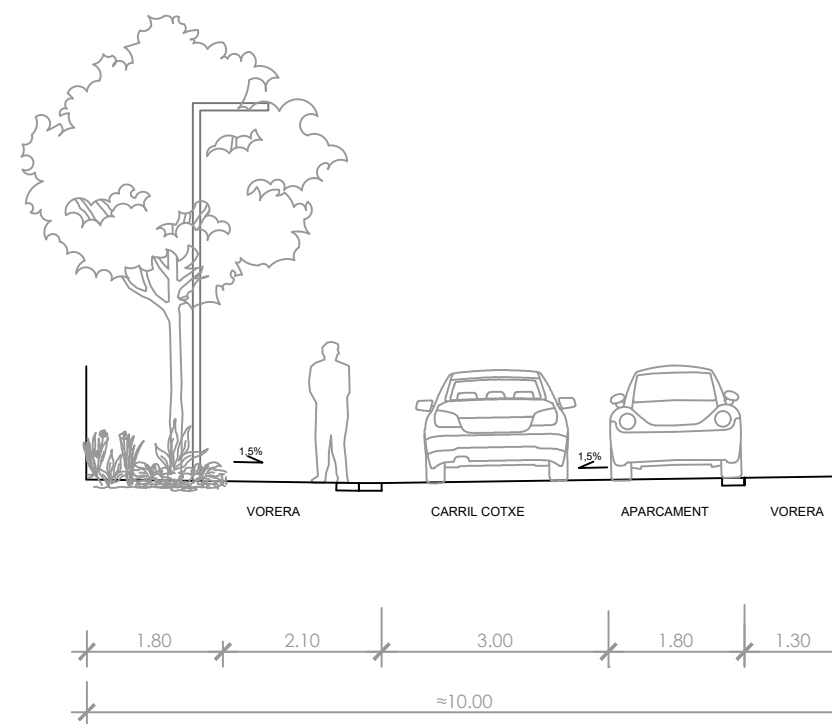
SECCIÓ PROPOSTA CARRER
