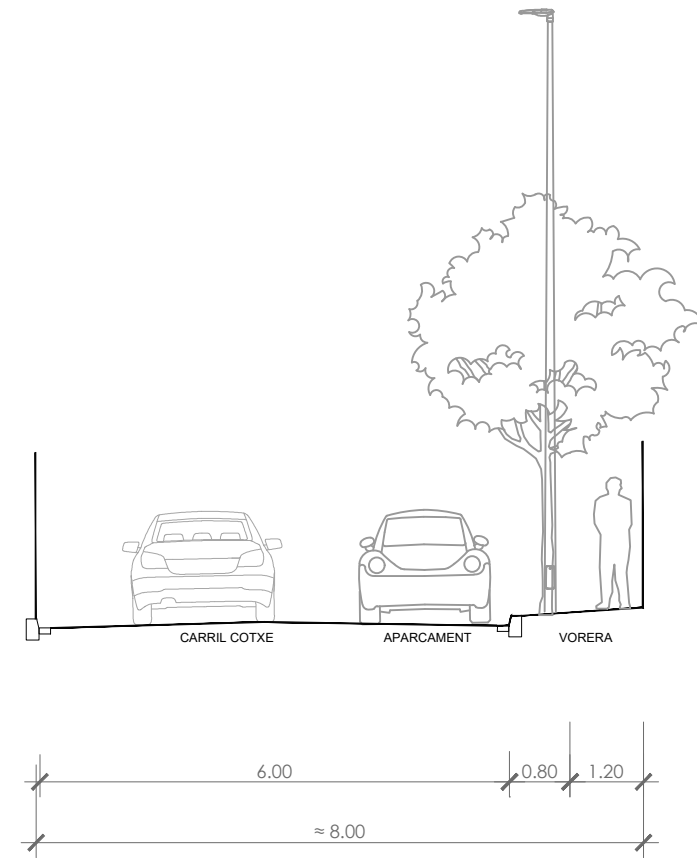
SECCIÓ ESTAT ACTUAL CARRER
