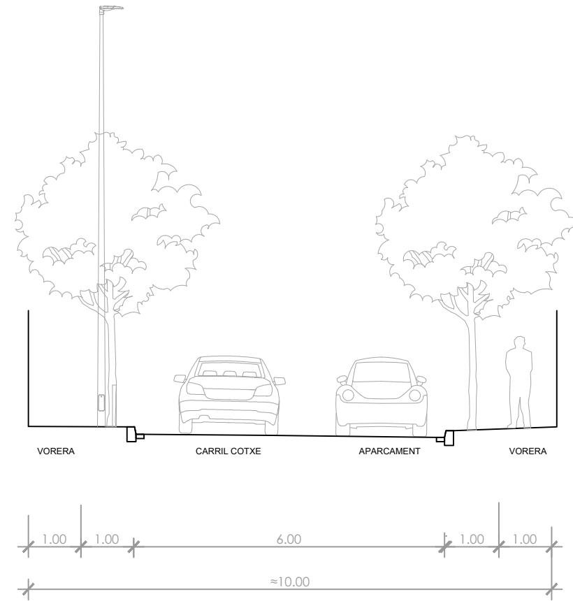
SECCIÓ ESTAT ACTUAL CARRER
