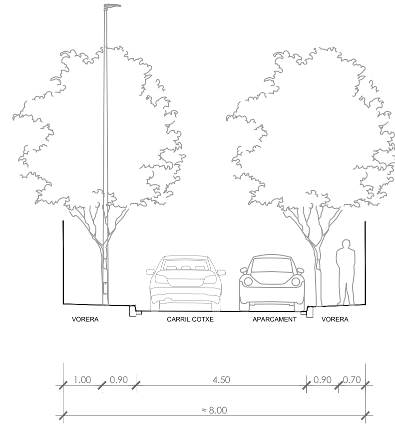
SECCIÓ ESTAT ACTUAL CARRER
